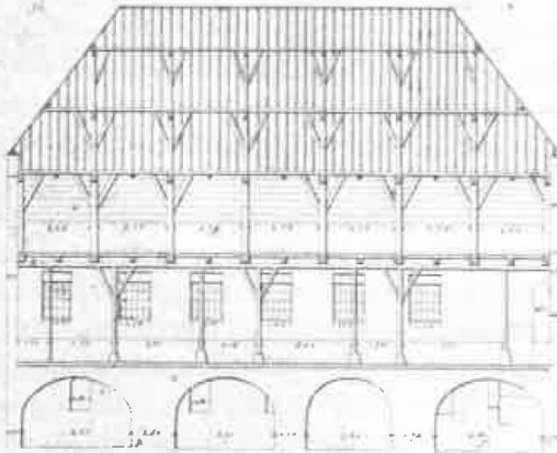
44. Opmetingstekening van de grote schuur uit 1514. Langsdoersnede, 1862.
